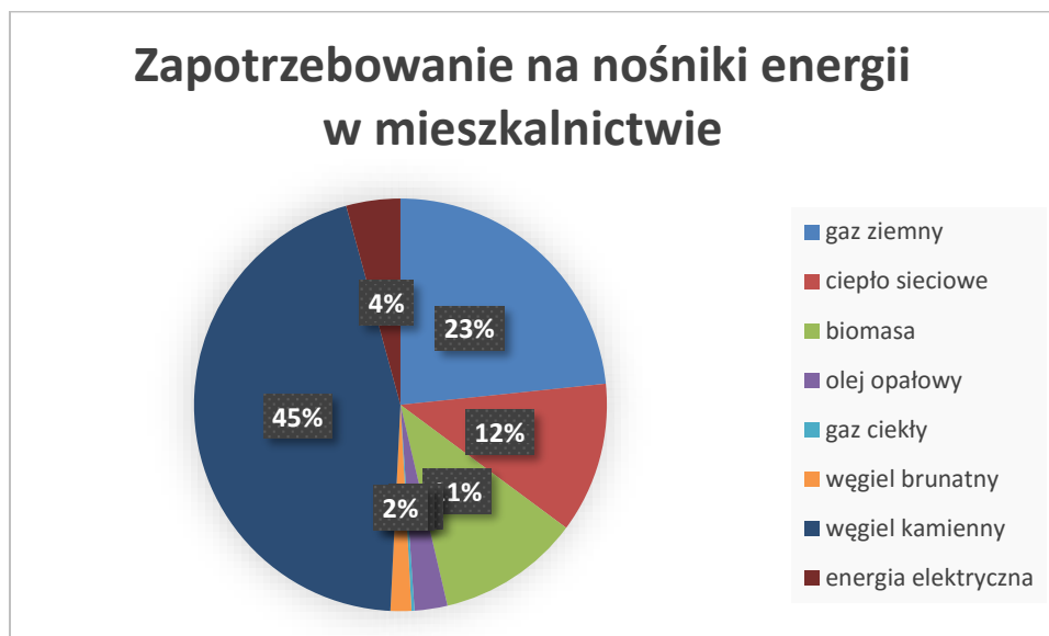
Rys. 4 Struktura pokrycia zapotrzebowania na ciepło w sektorze mieszkaniowym w mieście Żary
